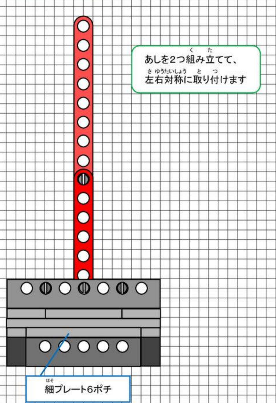
オから見た図
