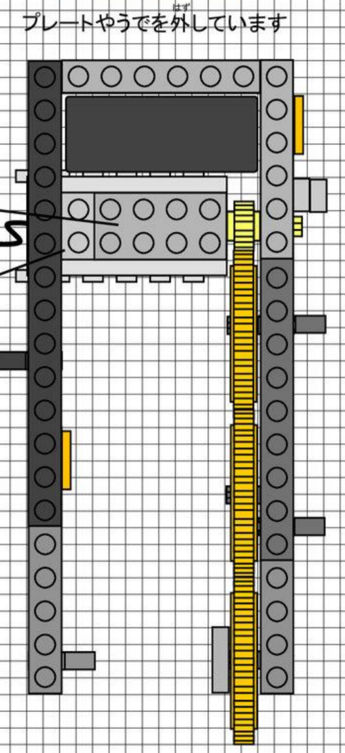
エから見た図
