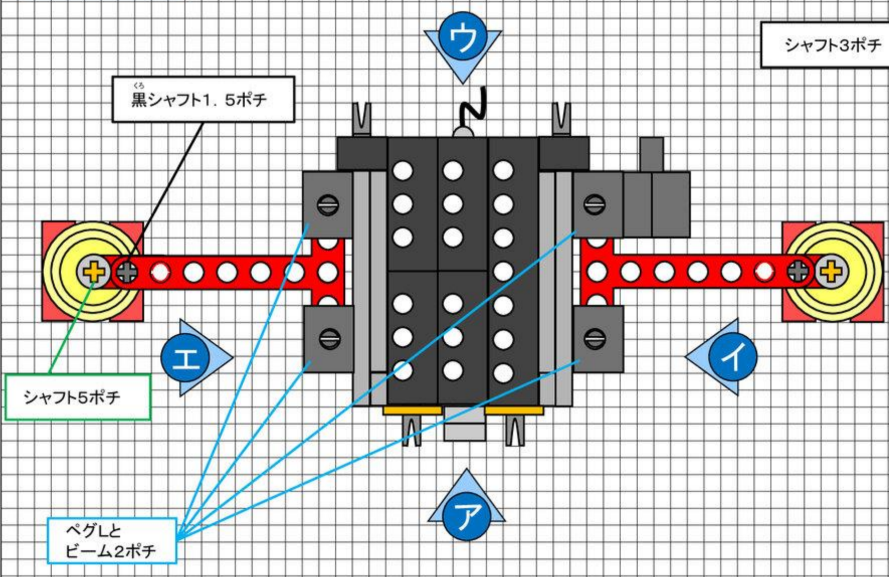
上から見た図
