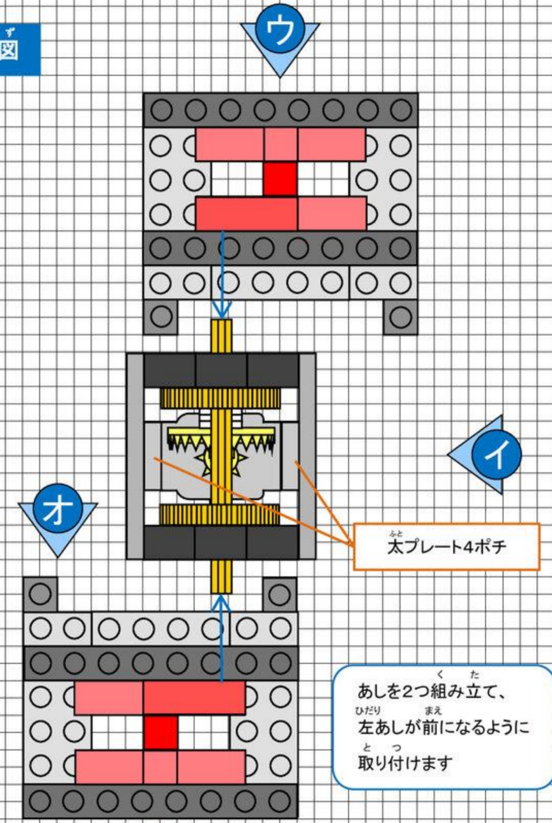
下から見た図
