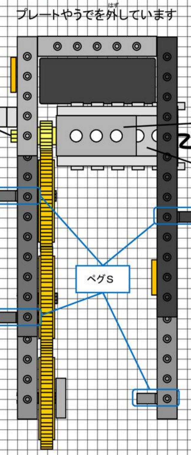
イから見た図
