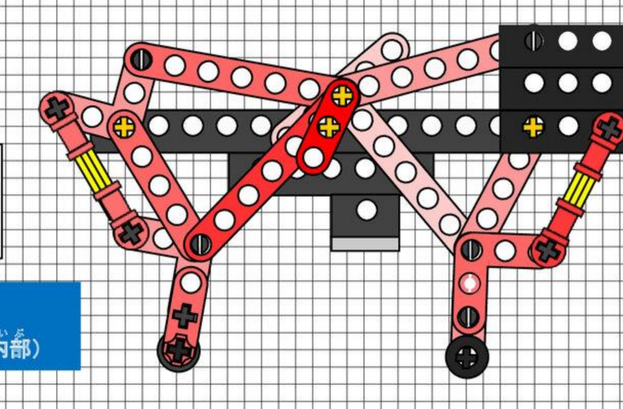
ウから見た図 (手前のビームを外した内部)
