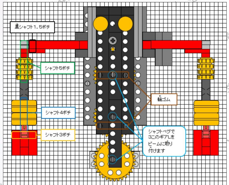
[図面(部分)]
